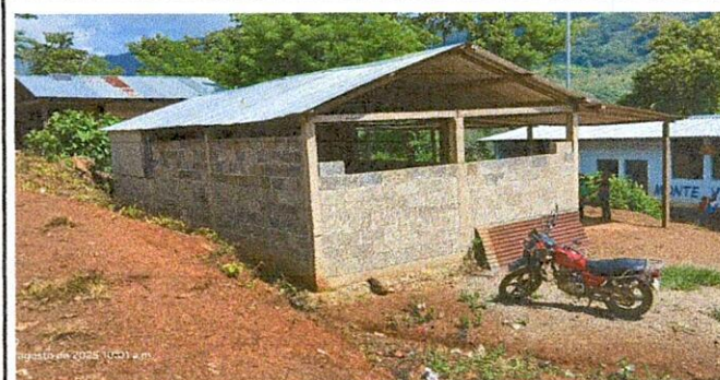
Foto: 4 INSTALACIÓN DE ESTRUCTURA MÓDULO 2
